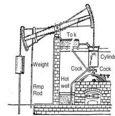
ਚਿਤਰ 5: ਨਿਊ ਕਮਨ ਦਾ ਇੰਜਣ
