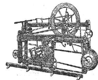
ਚਿੱਤਰ 3: ਕ੍ਰੌਮਪਟਨ ਦਾ ਮਯੂਲ
